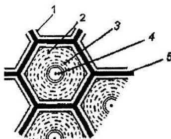
18-rasm. Tanho tolaning ko'ndalang kesimi.
