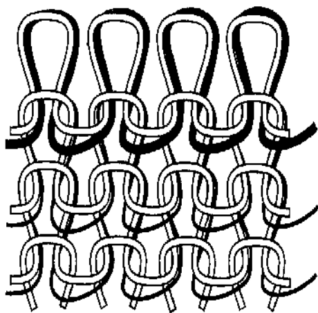
66-rasm. Plyush to'qimasi tuzilishi.
