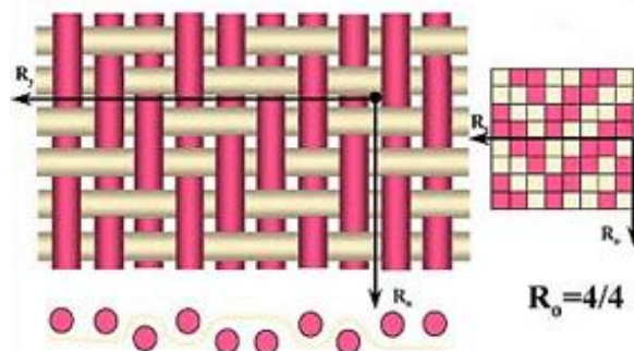
56-rasm. Teskari sarja o'rilishi.
