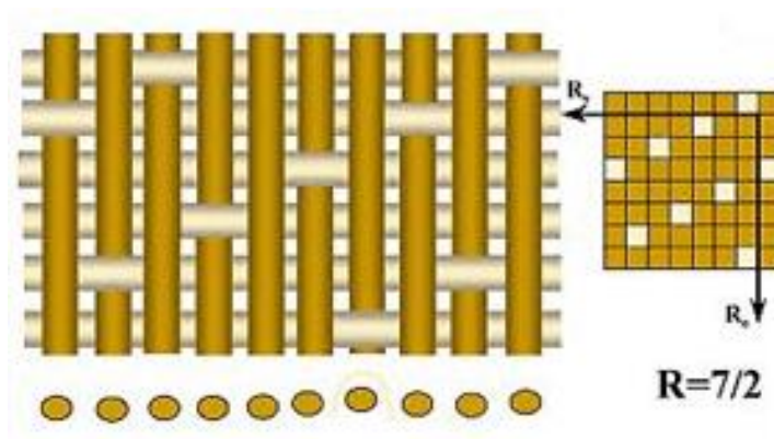
52-rasm. Atlas o'rilishi.
