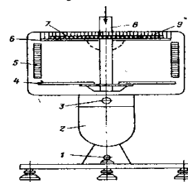
75-rasm. PT-2 uskunaning shakli.
